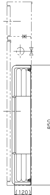
側面図
