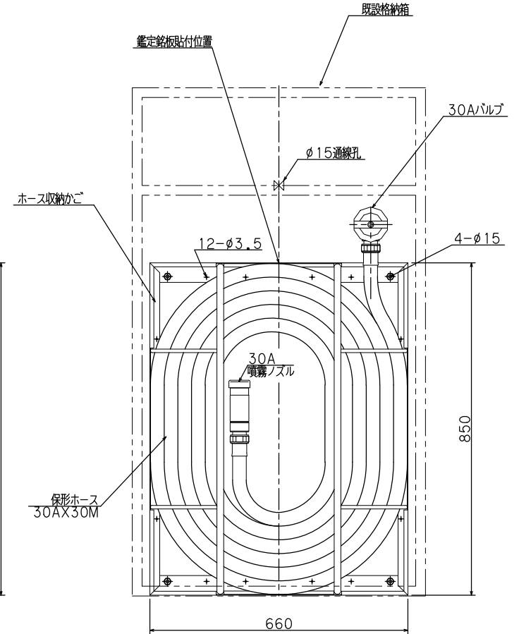
内部格納図
