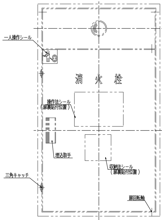
正面図
