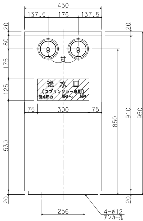
正面図
