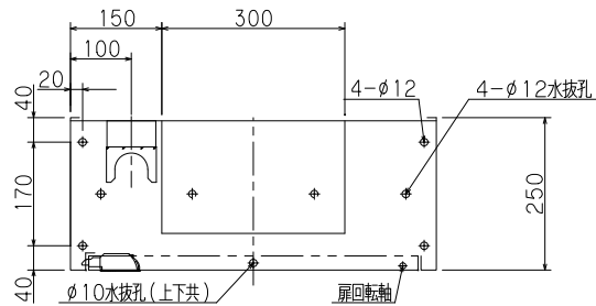
露出型
