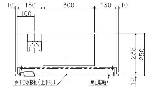
差込型
