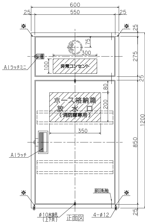
露出型
