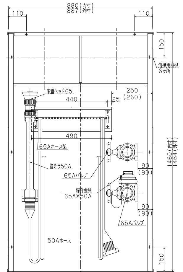
差込型内部格納図 (横配管の場合)
