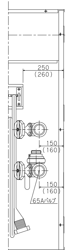
(裏配管の場合)
