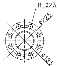
JIS20K-100A
