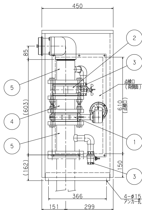
側面図
